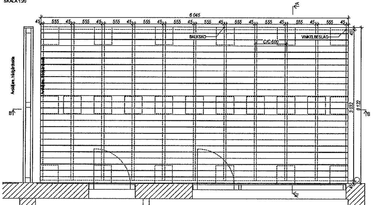
PLAN SKALA 1:20
