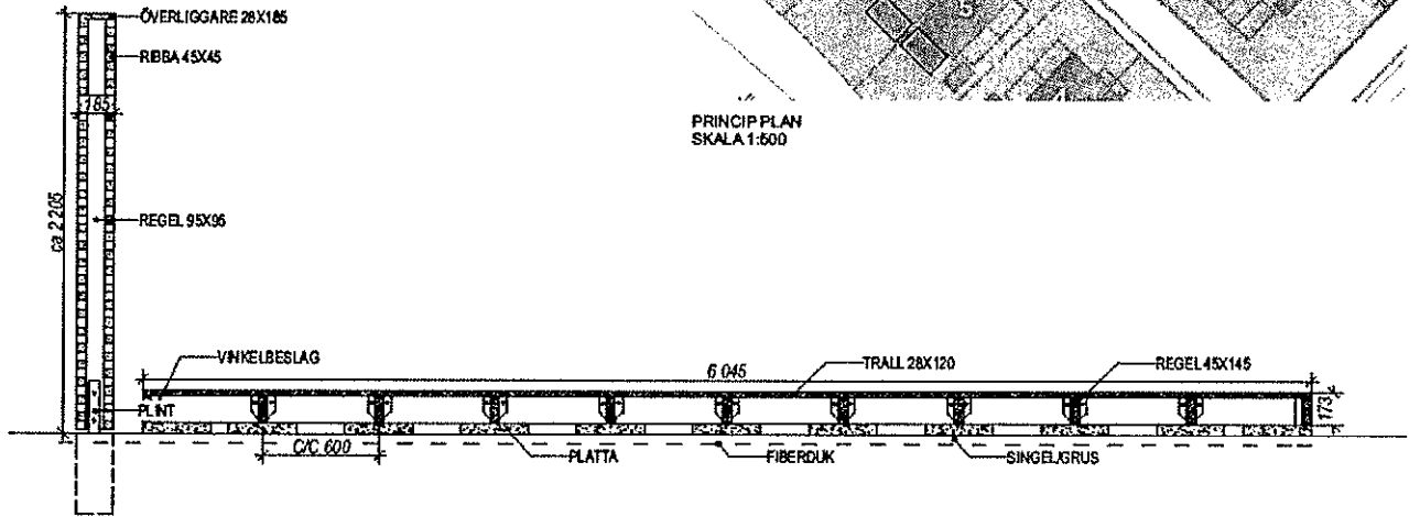
SEKTION B-B SKALA 1:20
