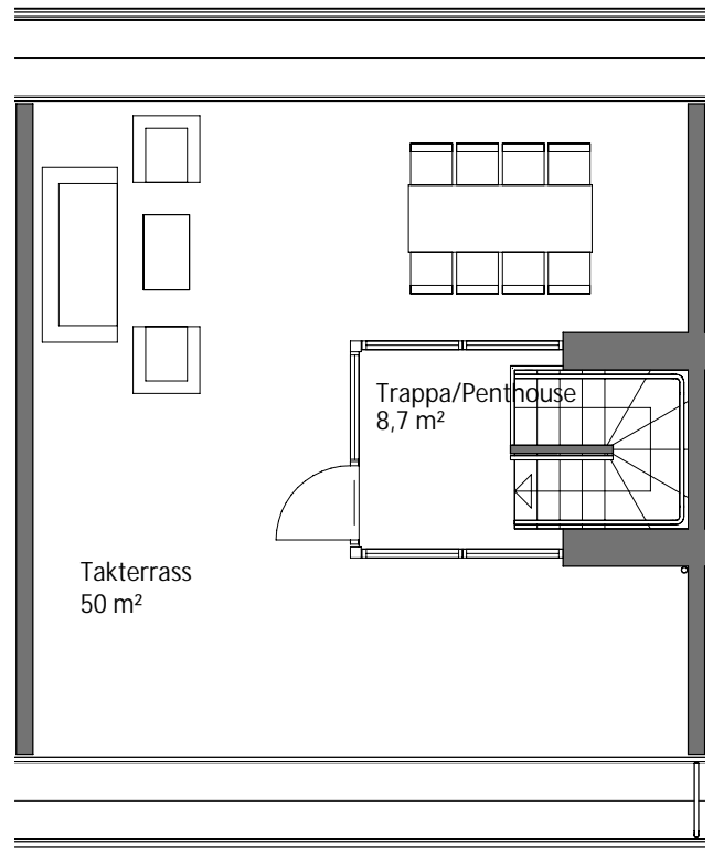
TAKPLAN
