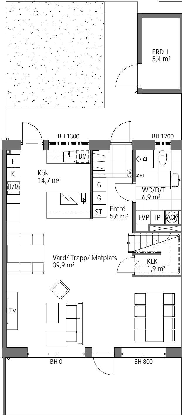
BOTTENVÅNING
