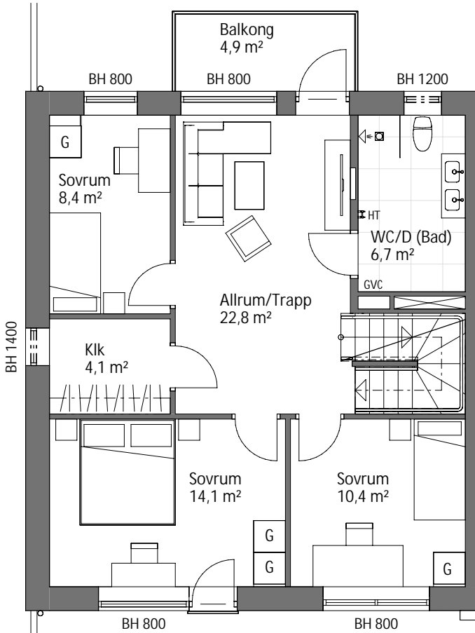
ÖVERVÅNING
