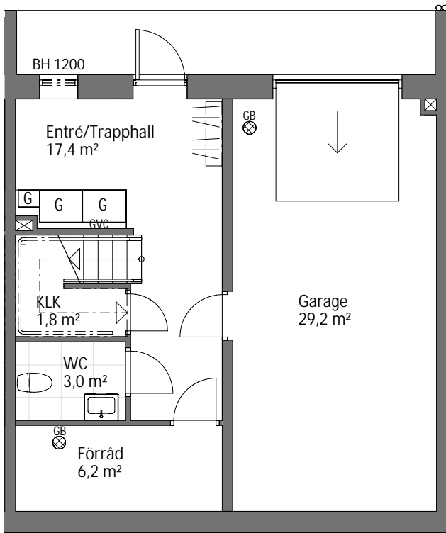
KÄLLARE
