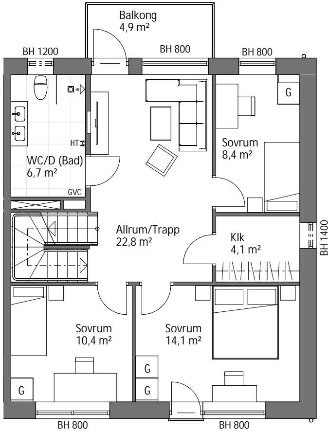
ÖVERVÅNING
