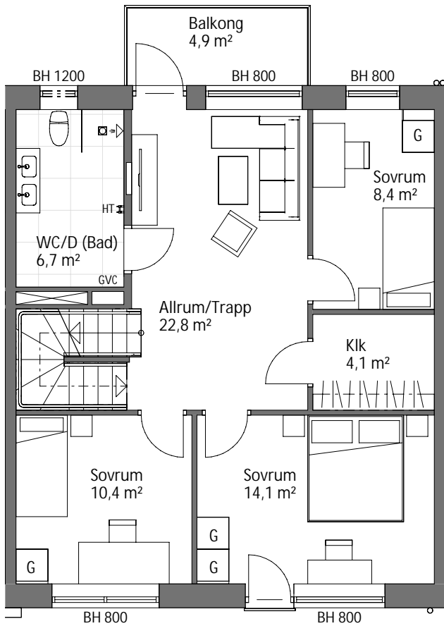
ÖVERVÅNING
